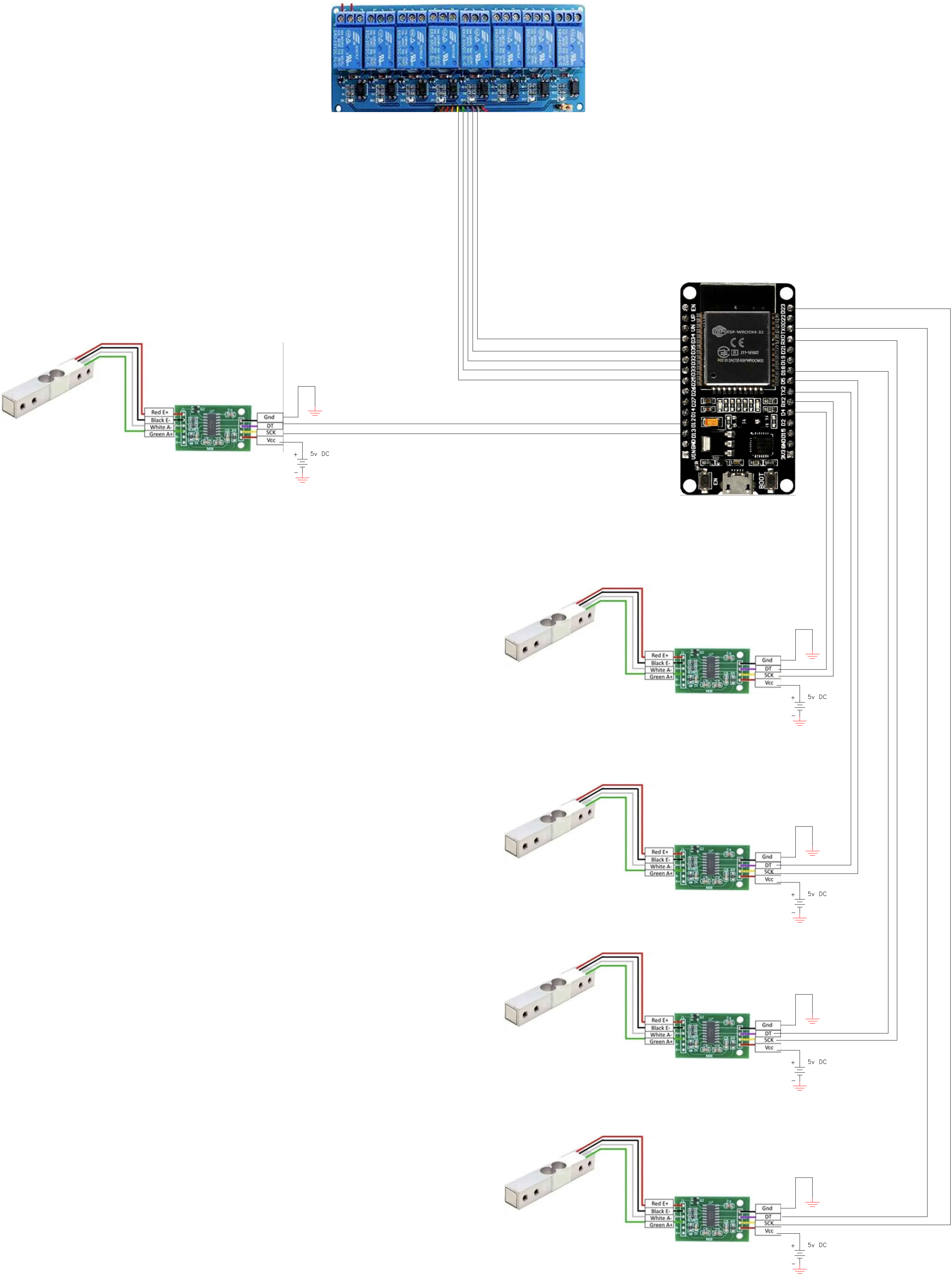
2 PLANO DE CONEXIONES
